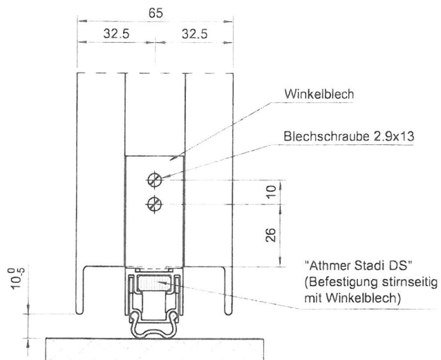
"Athmer Stadi Typ DS"
