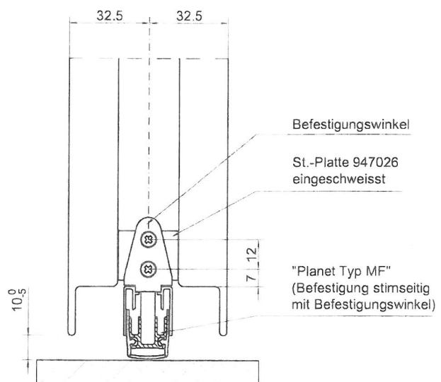
"Planet Typ MF"
