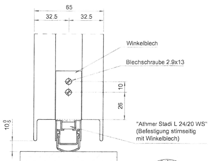
"Athmer Stadi Typ L 24/20 WS"
